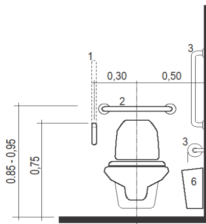
Σχήμα 84- Ύψη λεκάνης.
