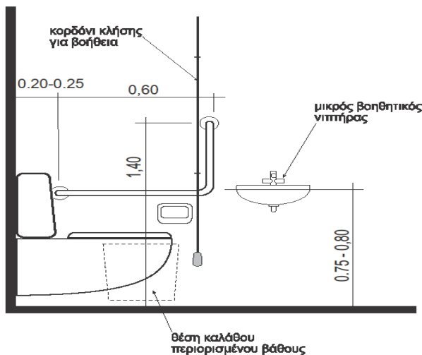
Σχήμα 87- Χειρολαβές χώρων υγιεινής.
