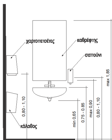
Σχήμα 91 - Διαμόρφωση νιπτήρα.
