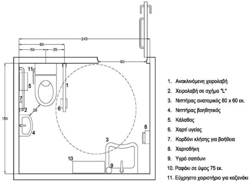
Σχήμα 83- Παράδειγμα διαμόρφωσης χώρου υγιεινής τύπου A με ελάχιστη διάσταση 1,85μ (1,80μ καθαρή διάσταση).
