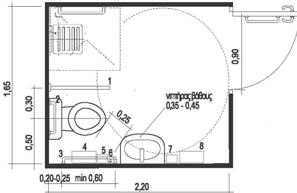
Σχήμα 97- Χώρος υγιεινής τύπου B με ισόπεδο ντους, για νοσοκομεία και χώρους διαμονής ασθενών.
