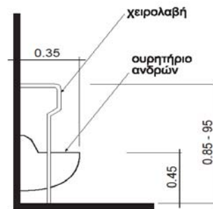
Σχήμα 80- Ουρητήρας χρήση αναπηρικού τροχοκαθίσματος.
