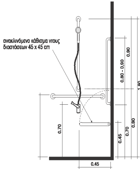
Σχήμα 96- Εξοπλισμός χώρου ντους.
