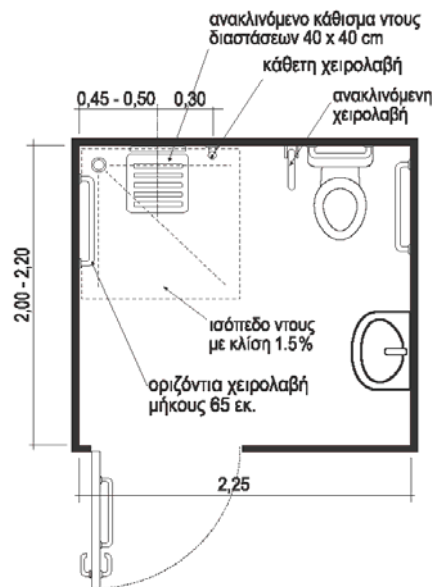
Σχήμα 95 - Παράδειγμα χώρου υγιεινής με ισόπεδο ντους.
