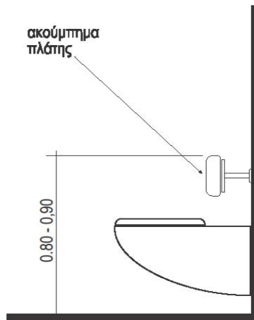
Σχήμα 85- Πλάγια όψη λεκάνης με εντοιχισμένο καζανάκι και με ακούμπημα πλάτης.
