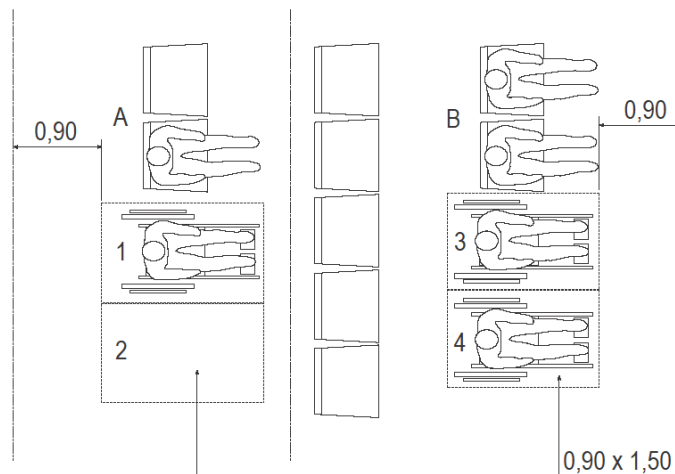
Σχήμα 67- Παράδειγμα διαμόρφωσης θέσεων για άτομα με μειωμένη κινητικότητα σε τροχόκαθισμα.
