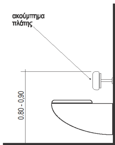
Σχήμα 79- Πλάγια όψη λεκάνης με εντοιχισμένο καζανάκι και με ακούμπημα πλάτης.
