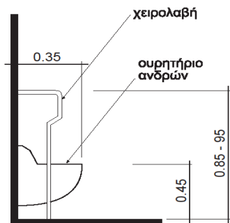
Σχήμα 74- Ουρητήρας χρήστη τροχοκαθίσματος.
