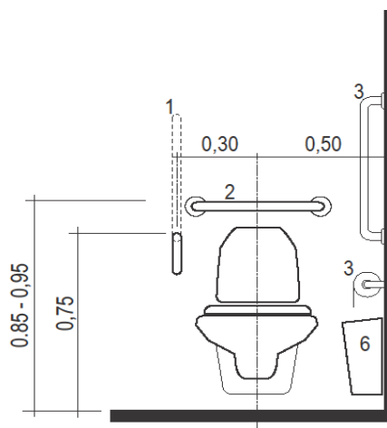
Σχήμα 78- Παράδειγμα όψης λεκάνης.
