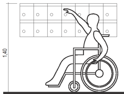
Σχήμα 7- Ύψος τοποθέτησης θυρίδων.
