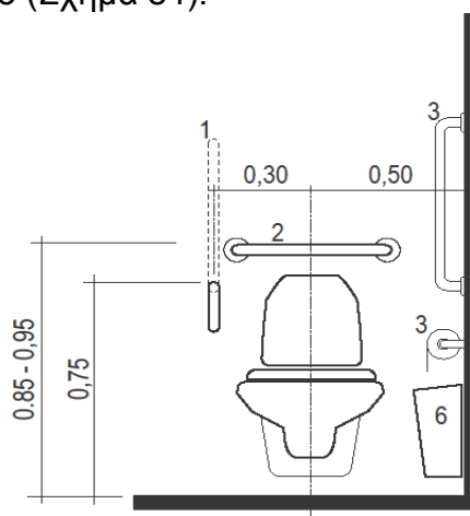
Σχήμα 84 – Όψη λεκάνης.
